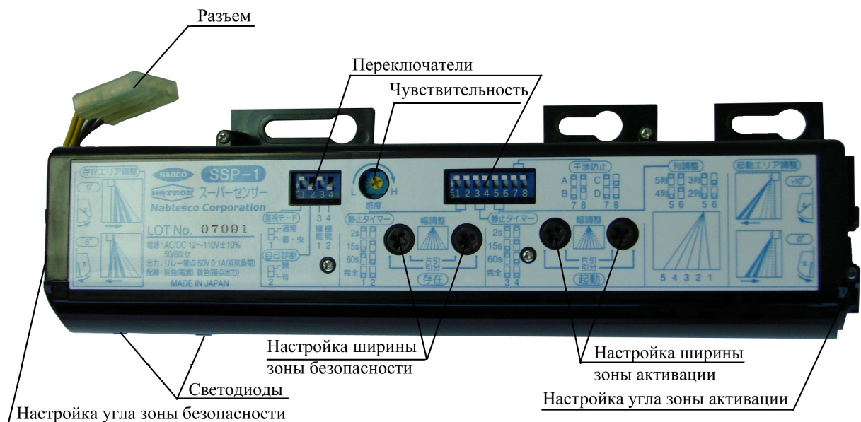
Вид сенсора без кожуха
